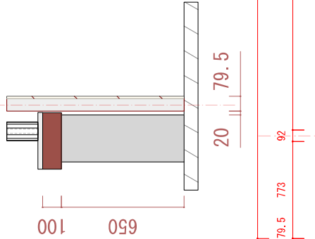
断面図 S=1/20
