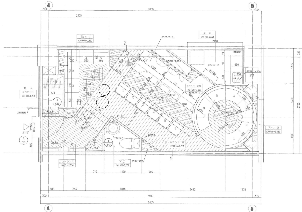
第20桂和ビル5階4号 平面図
