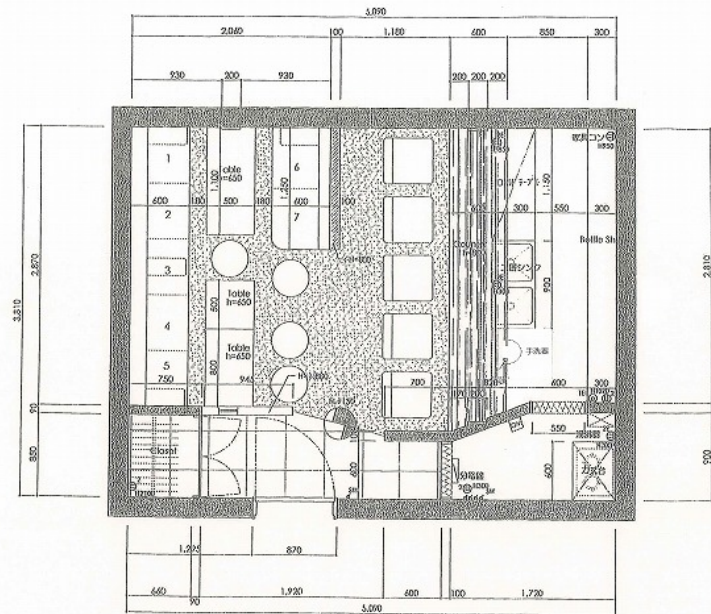
ニュー桂和ビル7階12号 平面図
